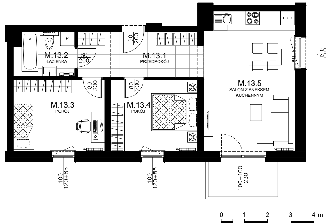
Budynek B3, mieszkanie M.13 3 - pokojowe
